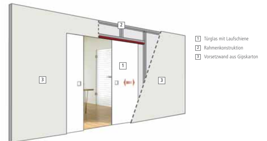
Schiebesystem 2-flügelig
